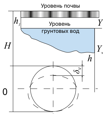
Рисунок 6. Схема прокладки трубы в грунте
